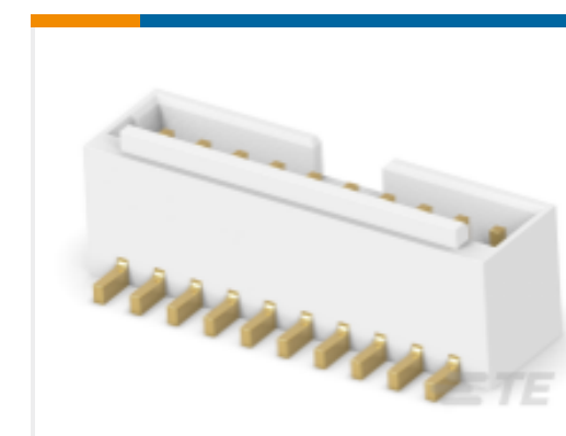
TE Part # 3-2380320-0 1.5P 10POS WTB VERT BRD W LATCH AU NAT
