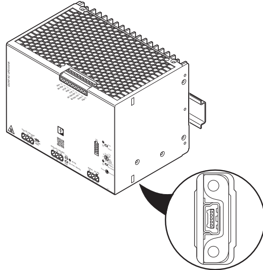
Figure 15 Service USB interface Mini type B (device bottom) (5.1)
