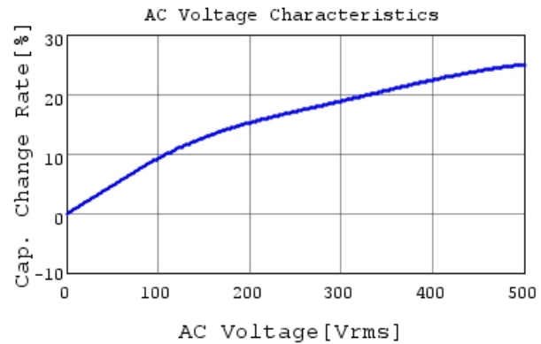
DE1B3RA681KN4AQ01F C-AC Voltage capchange, I
