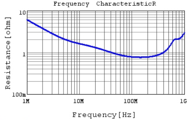
DE1B3RA681KN4AQ01F R DCOV, 20degC
