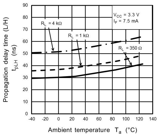
Fig. 12.2.17 t_{pLH} - T_a
