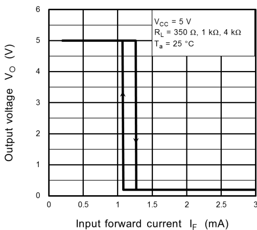
Fig. 12.2.5 V_O - I_F
