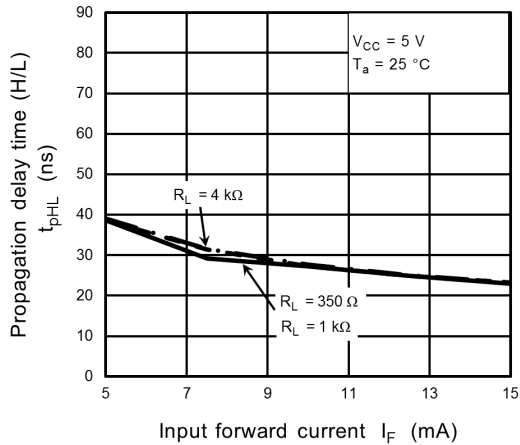
Fig. 12.2.19 t_{pHL} - I_F
