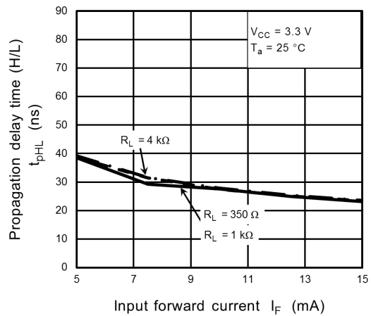
Fig. 12.2.22 t_{pHL} - I_F
