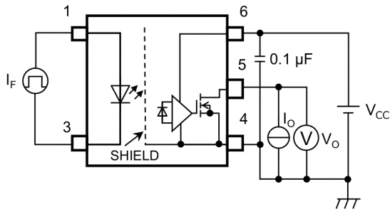
Fig. 12.1.5 I_{FHL} , I_{FLH} , I_{HYS} Test Circuit
