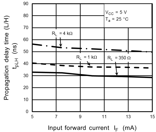
Fig. 12.2.20 t_{pLH} - I_F
