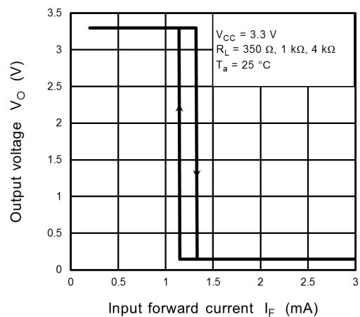
Fig. 12.2.6 V_O - I_F
