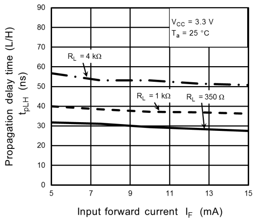
Fig. 12.2.23 t_{pLH} - I_F
