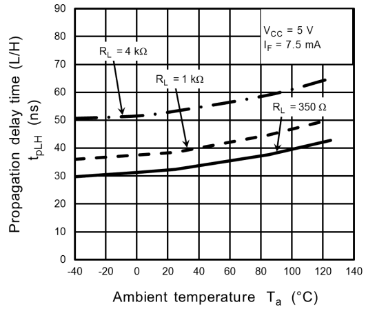
Fig. 12.2.14 t_{pLH} - T_a
