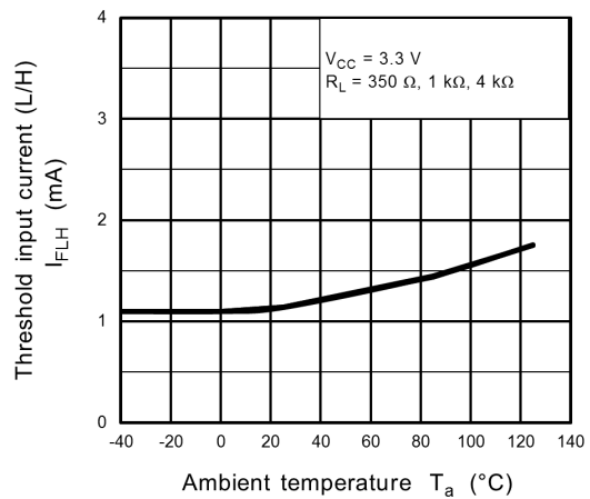
Fig. 12.2.10 I_{FLH} - T_a
