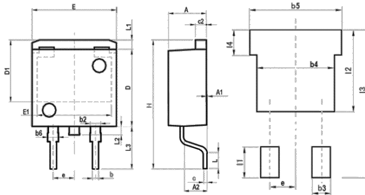
TO-263L, [-], (TO-263L)
