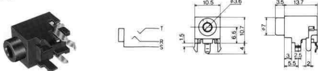
No.MX-362GL (φ3.5) STEREO
