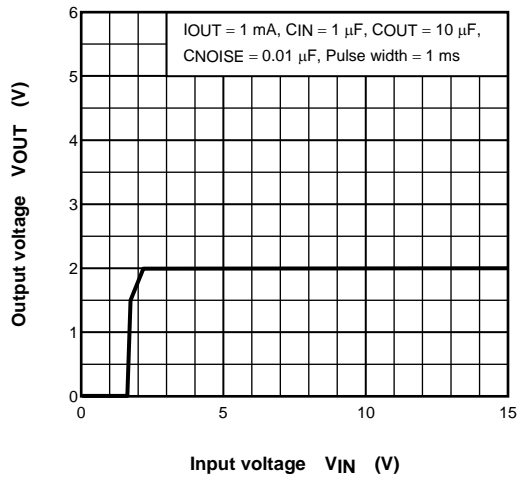
(TAR5SB20) V_{OUT} - V_{IN}
