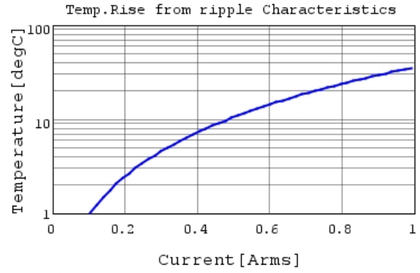
GRM033C80J104ME15 Temp.rise 800kHz
