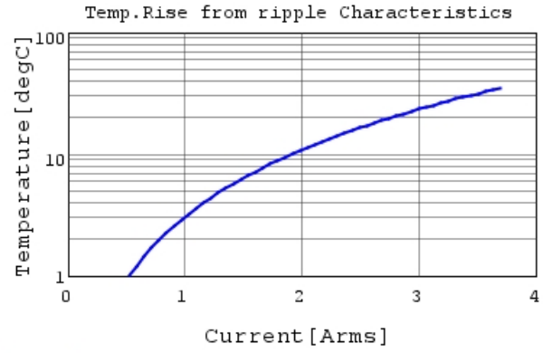
GRM035C80J225ME01 Temp.rise 1MHz
