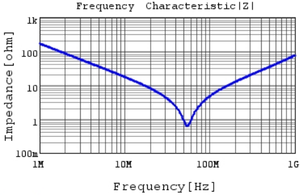
DE2E3SA102MJ3BX02F |Z| DCOV, 20degC
