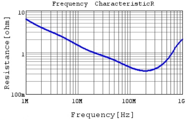
DE2E3SA102MJ3BX02F R DCOV, 20degC
