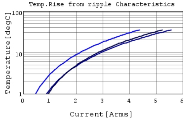
GRM188R60J226MEA0 Temp.rise — 80kHz
