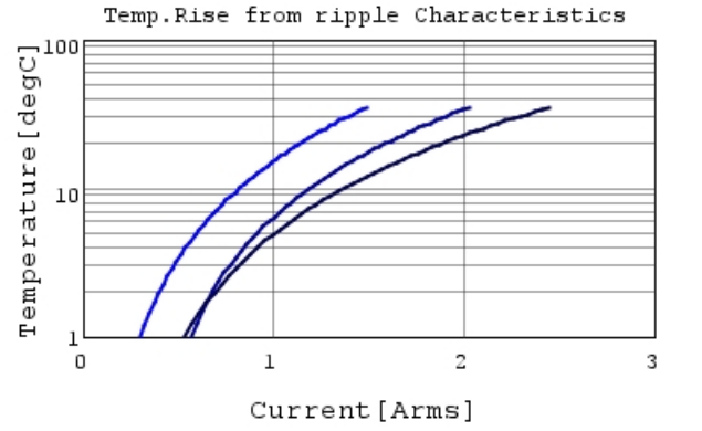
GCM188R71H224KA64 Temp.rise — 300kHz —
