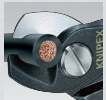
Kabelschnitt mit Kabelschneider: leichter, sauberer Schnitt ohne Verformung des Kabels
