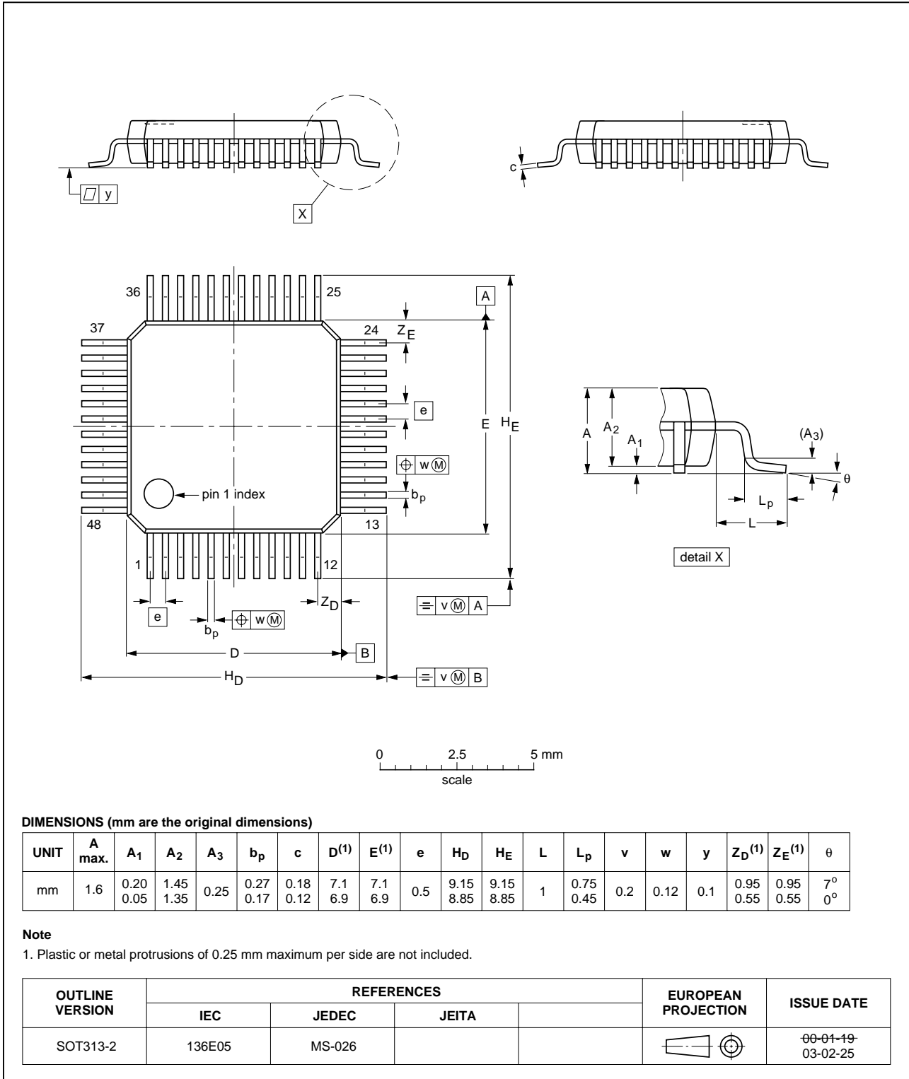
Fig 7. SOT313-2
