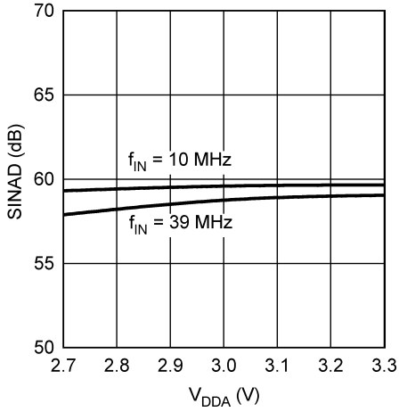
SINAD vs. V_{DDA}
