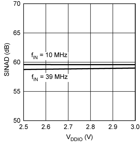
SINAD vs. V_{DDIO}
