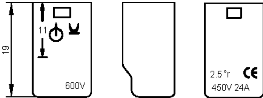
Dimensions : Millimetres
