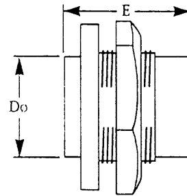
Universal Flange Receptacle
