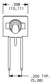
Actuator Shown In Pos. 1
