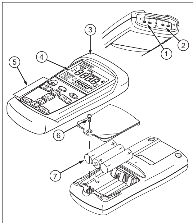
图 1. 部件
