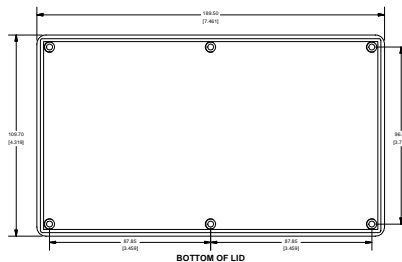
BOTTOM OF LID
