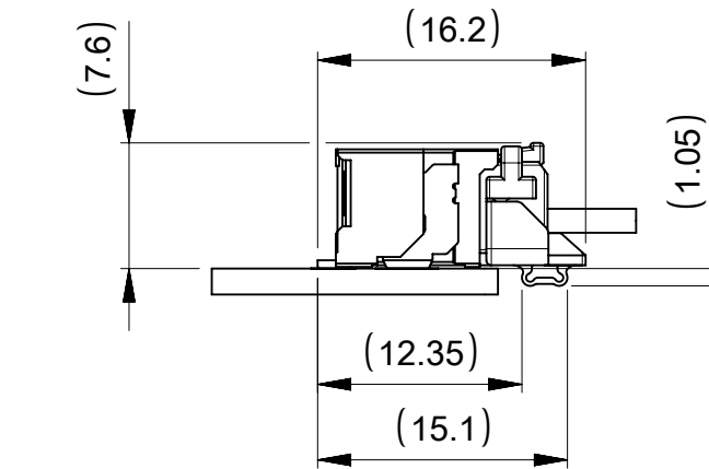
ISLタイプ嵌合図 MATED CONNECTORES OF ISL TYPE
