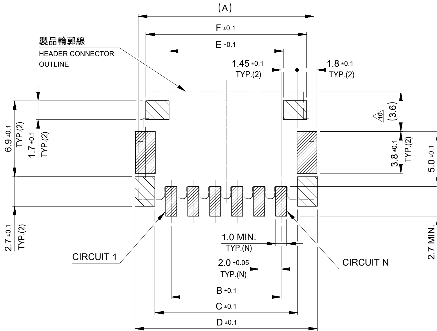
製品レイアウト PRODUCT LAYOUT
