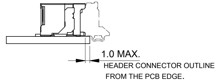
ISLタイプ基板レイアウトの注意点 PCB LAYOUT PRECAUTIONS FOR ISL TYPE
