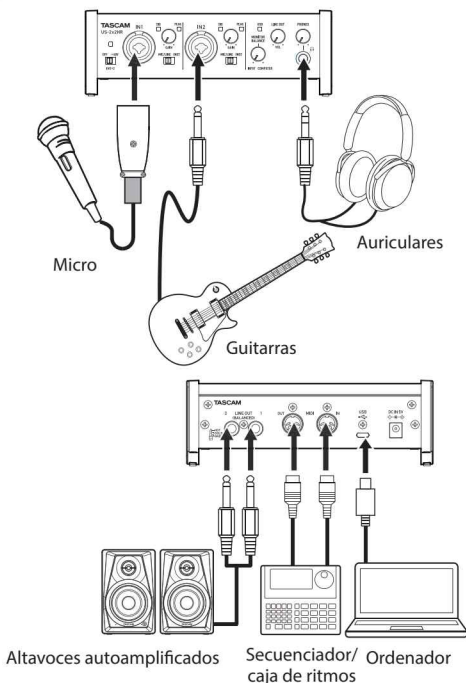
Ejemplos de conexión a un US-2x2HR
