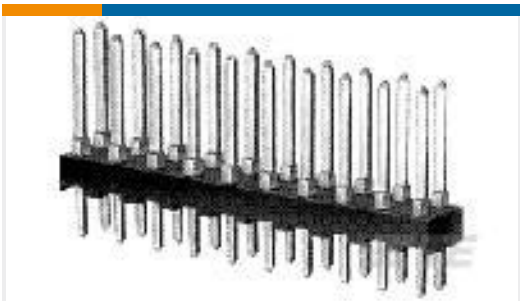
TE Part #3-87215-0 60 MODII HDR DRST UNSHRD .100
