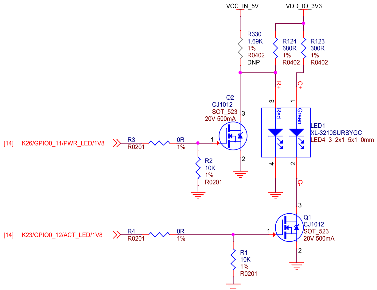
Fig. 3.57: BeagleY-AI LEDs
